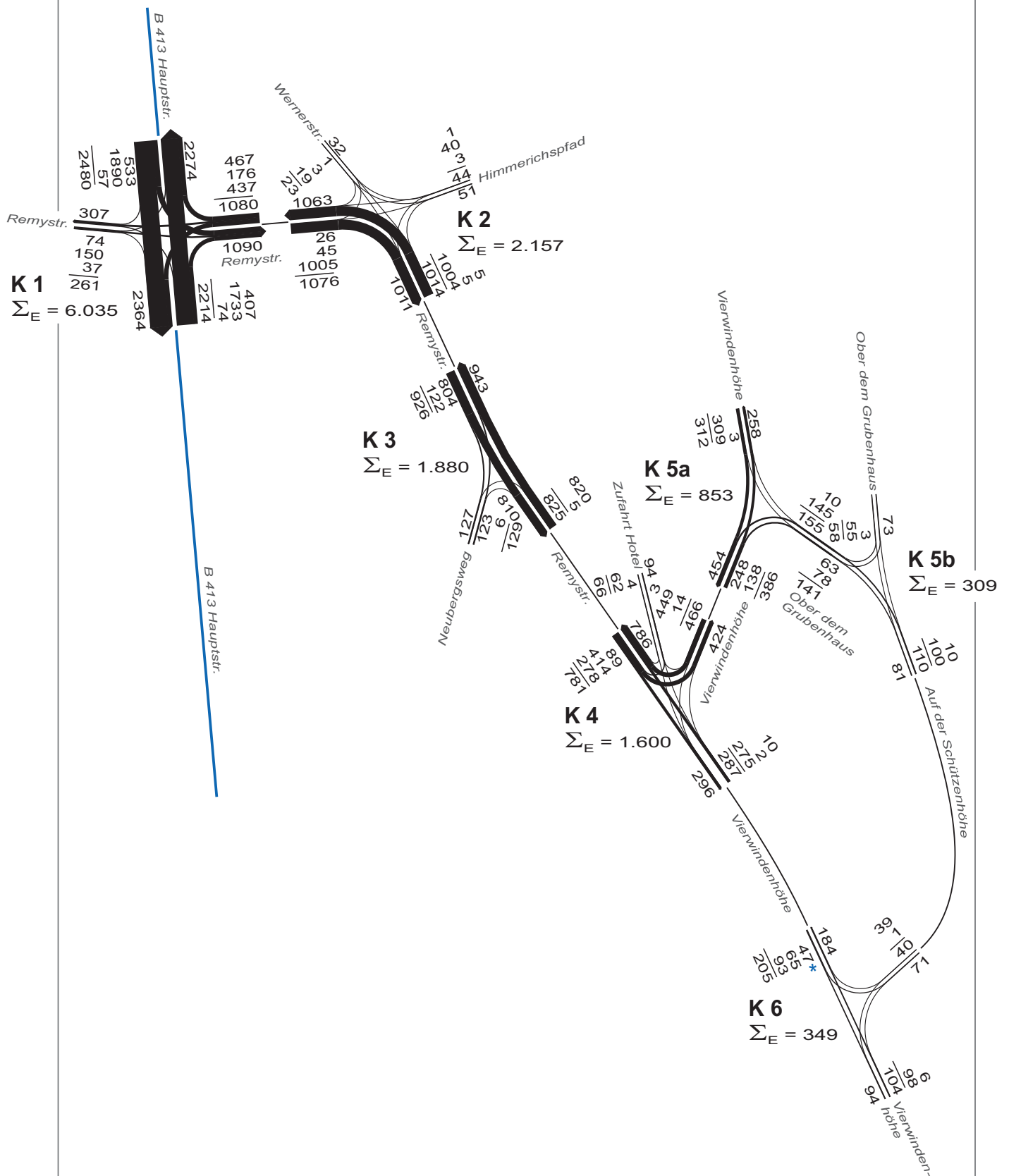
Abb. B3: Knotenstrombelastungen Gesamtverkehr 24h Dienstag 30.06.2020
