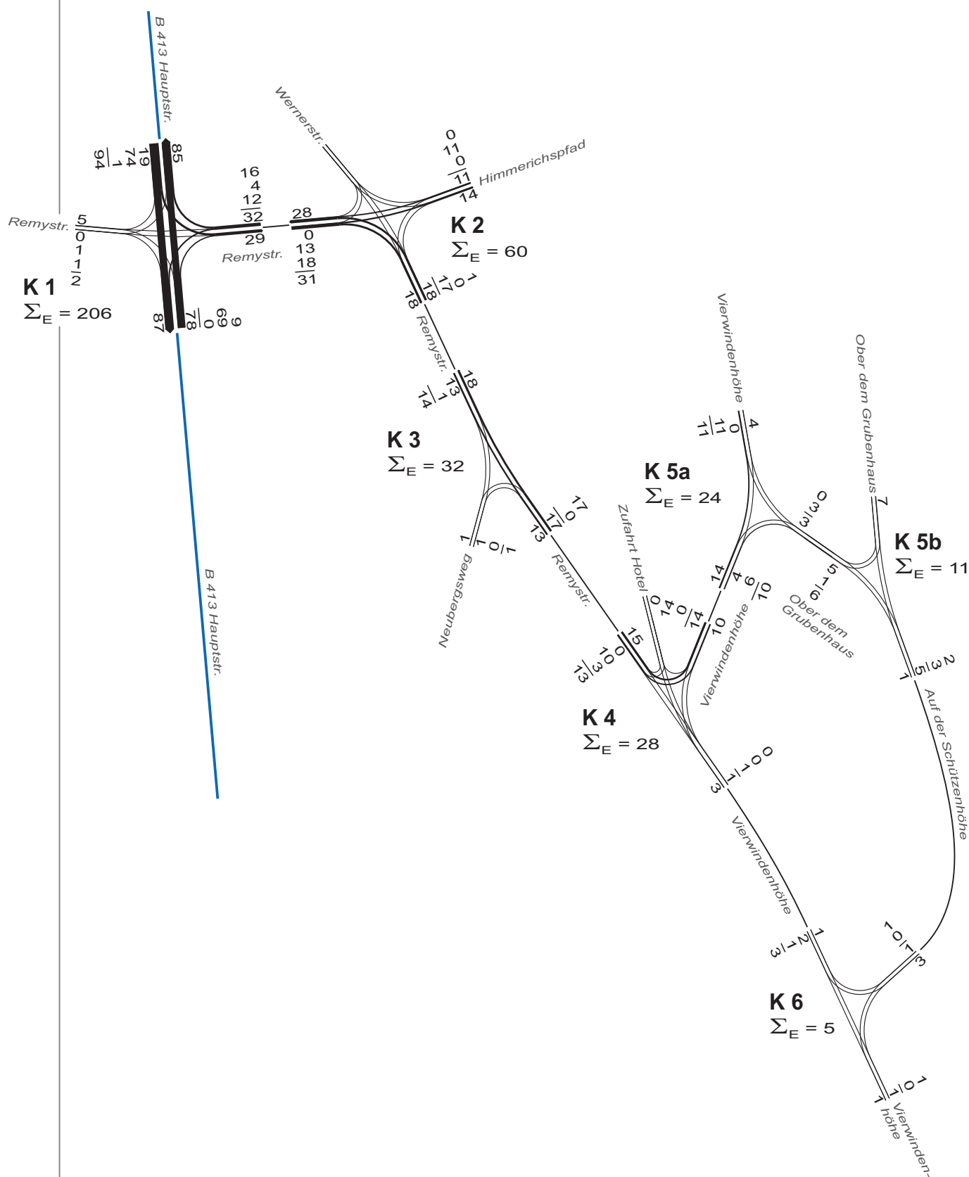
Abb. B4: Knotenstrombelastungen Schwerverkehr 24h Dienstag 30.06.2020
