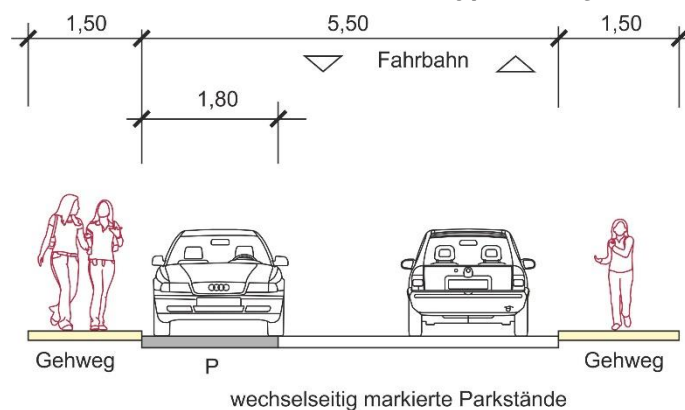
Typischer Querschnitt Vierwindenhöhe
