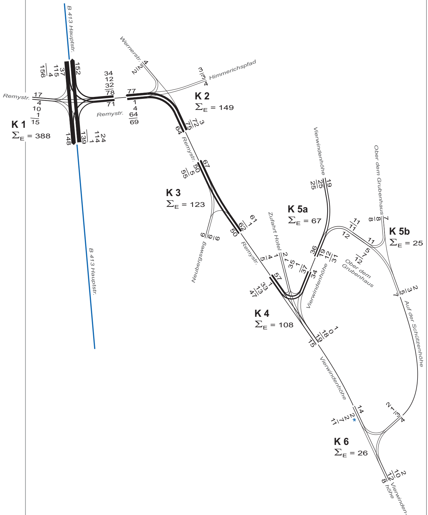
Abb. B5: Knotenstrombelastungen Gesamtverkehr Vormittagsspitzenstunde 10.30 - 11.30 Uhr Dienstag 30.06.2020
