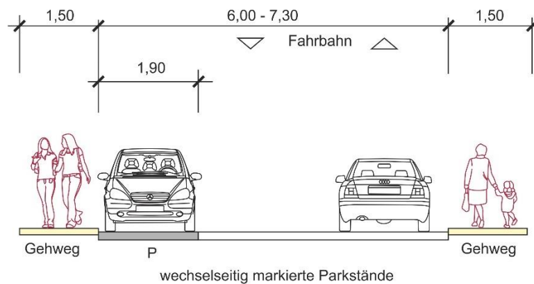
Bild B3 Typischer Querschnitt Remystraße
