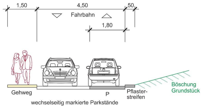
Typischer Querschnitt Auf der Schützenhöhe
