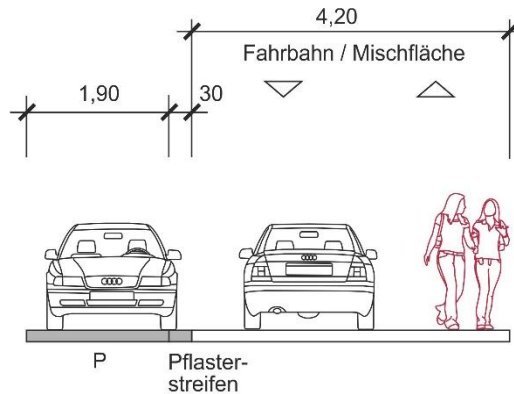
Typischer Querschnitt Ober dem Grubenhaus
