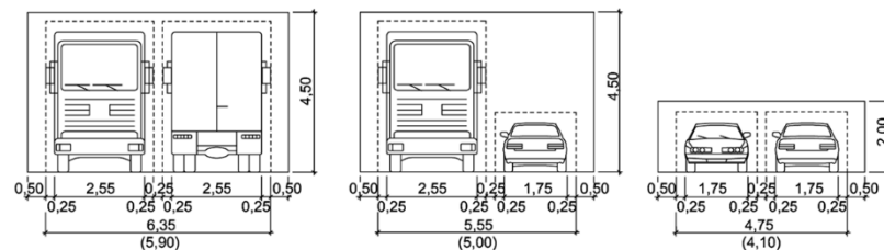
Bild B11 Verkehrsräume und lichte Räume beim Begegnen (Klammerwert mit eingeschränktem Bewegungsspielraum)
